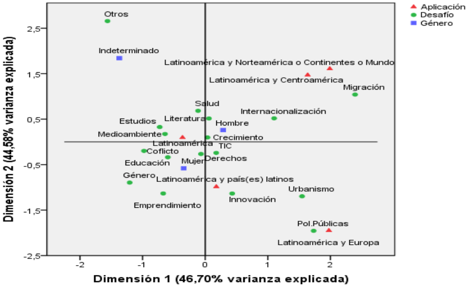
Figura 3 Gráfico de conjunto de puntos de categorías. Normalización principal por variable
